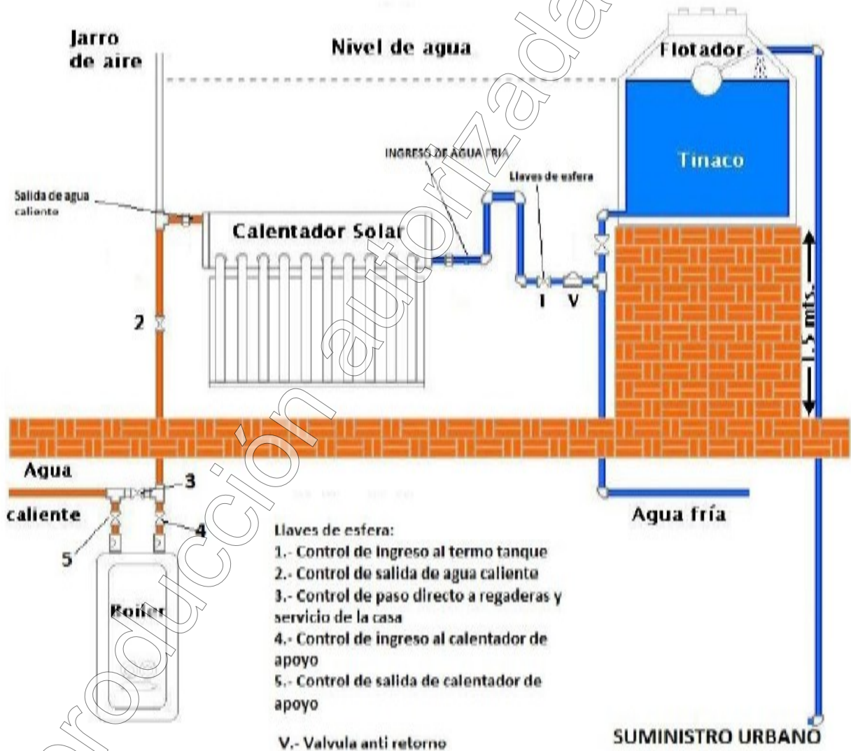
Figura 3 Instalación hidráulica
