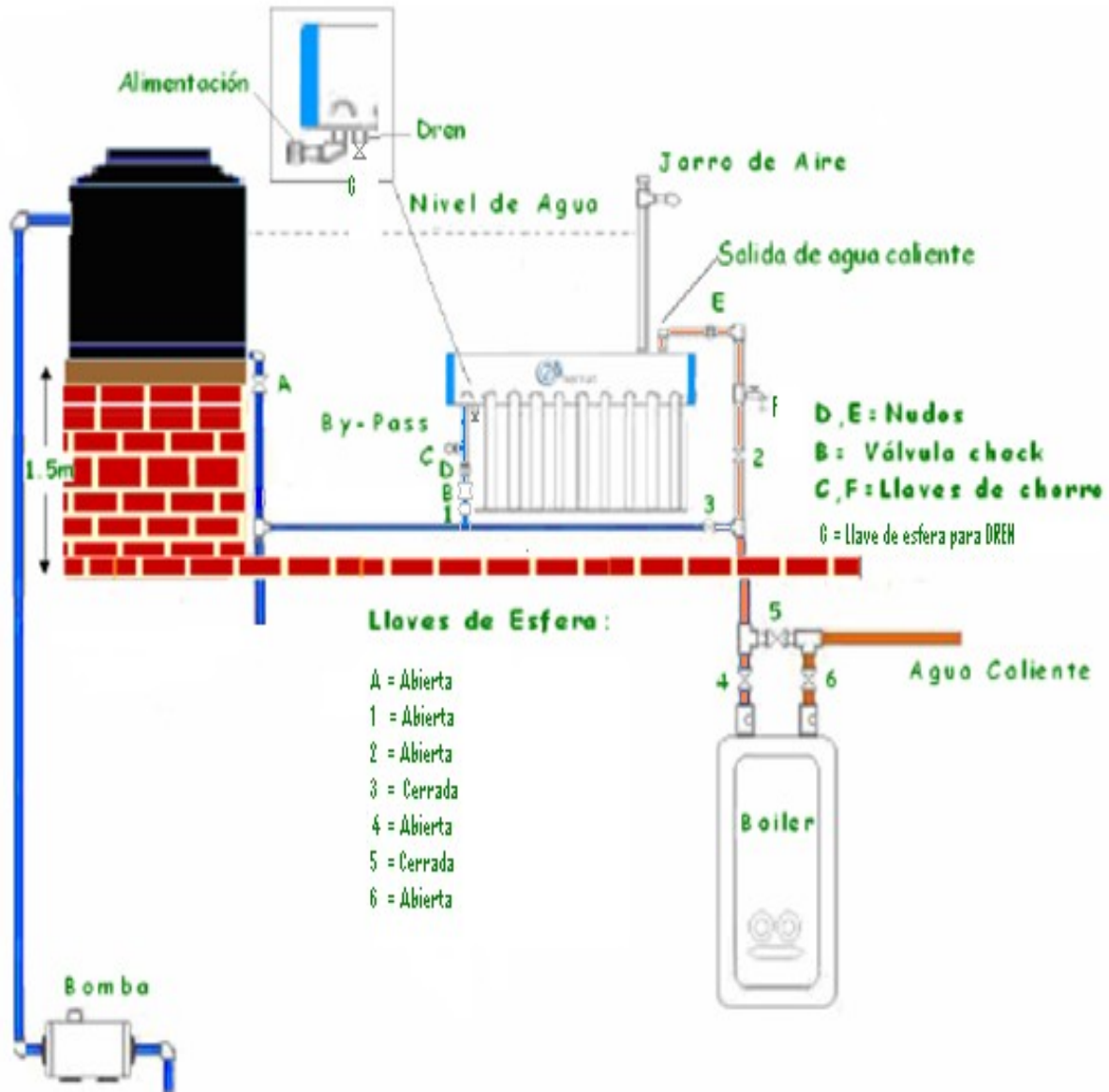
Figura 1 Instalación hidráulica con hidroneumático
