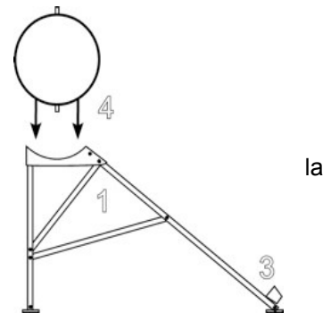
Figura 1 vista lateral de la estructura de soporte
