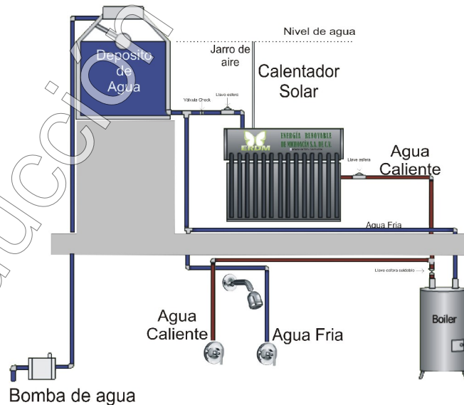
Diagrama de instalación hidráulica del “Calentador Solar”
