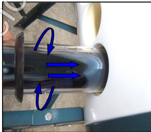
Figura 5 colocación de los tubos de vacío
