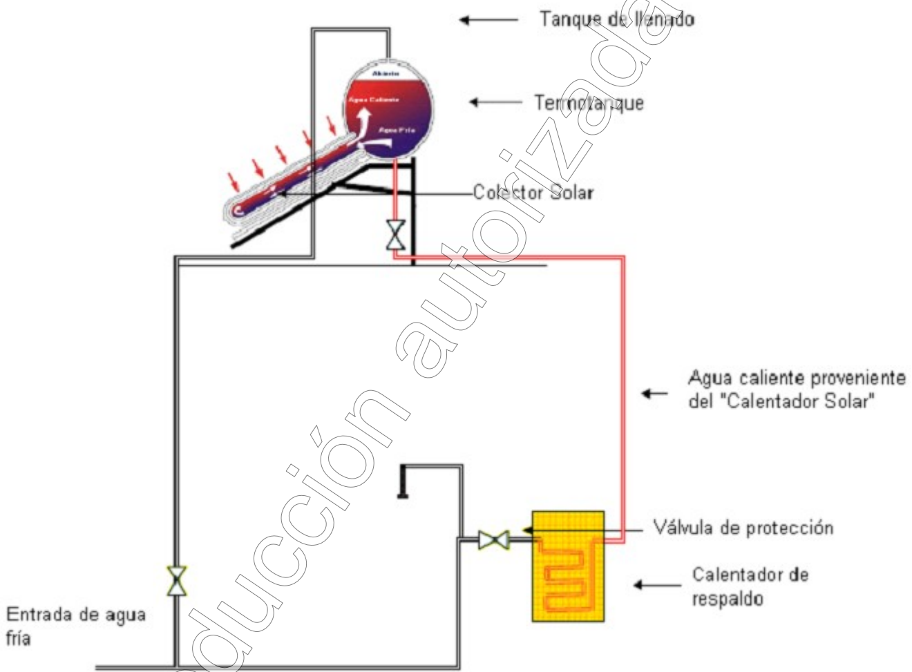
Figura 6 diagrama 1 instalación hidráulica del “Calentador Solar”
