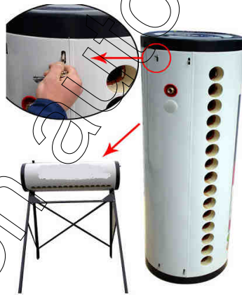
Figura 5 colocación del termostato en la estructura de soporte
