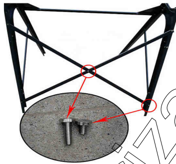
Figura 4 armado de la cruzeta trasera de la estructura de soporte
