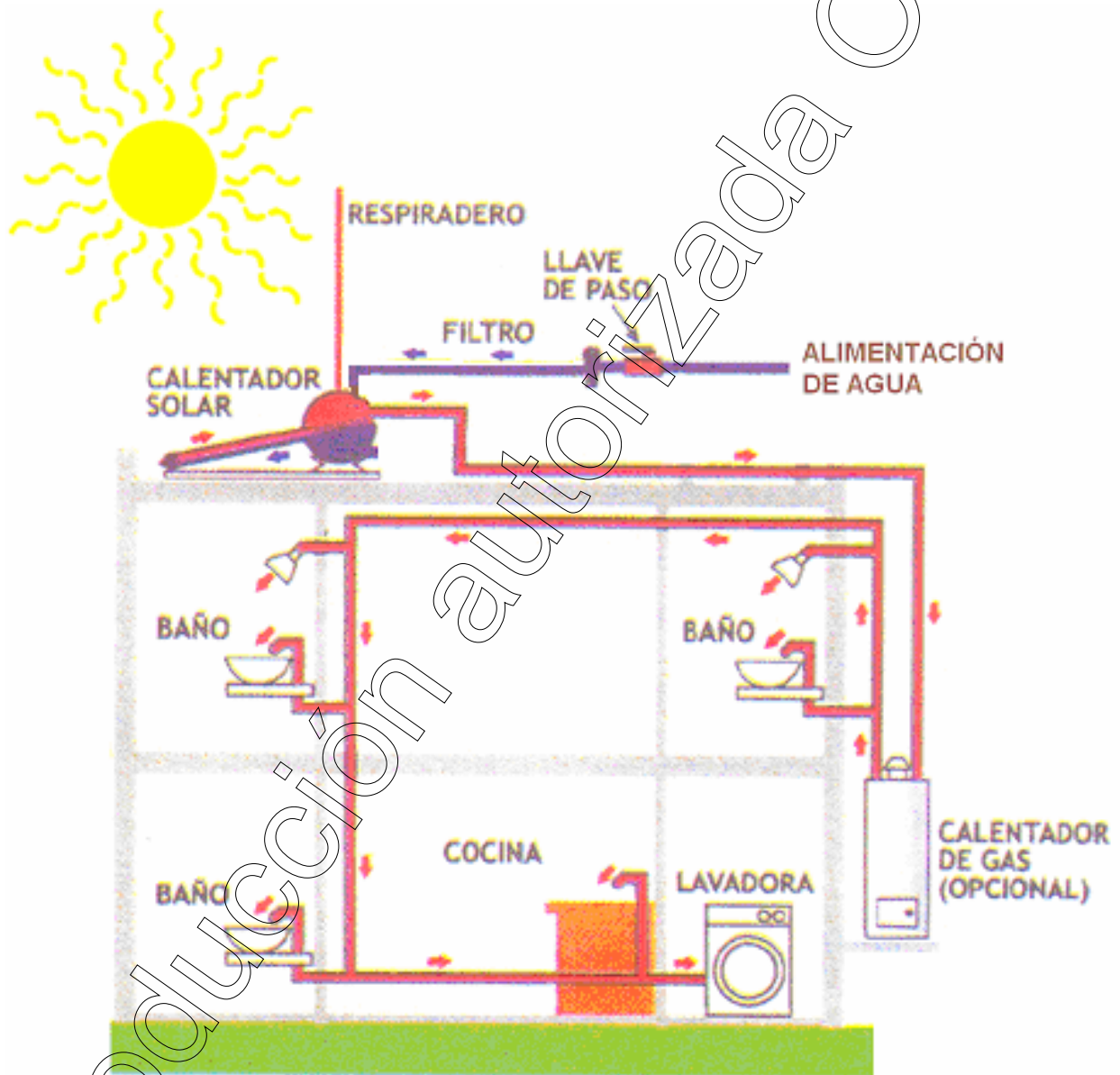
Figura 8 Instalación hidráulica del “Calentador Solar”
