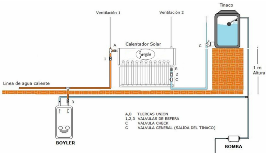
Figura 1 Instalación hidráulica
