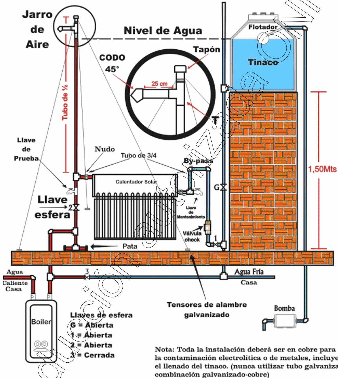
Figura 4 Instalación hidráulica
