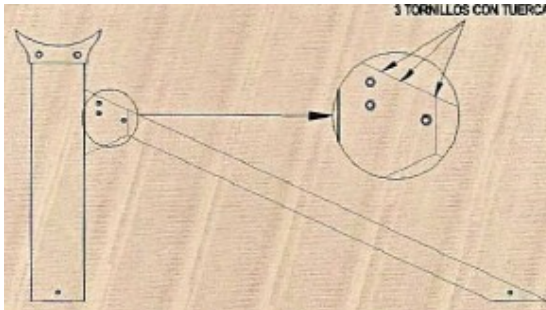
Figura 4 patas delanteras
