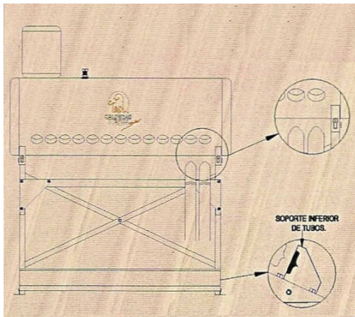
Figura 8 instalación de tubos de vacío
