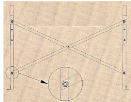
Figura 3 armado de soporte cruzado y patas
