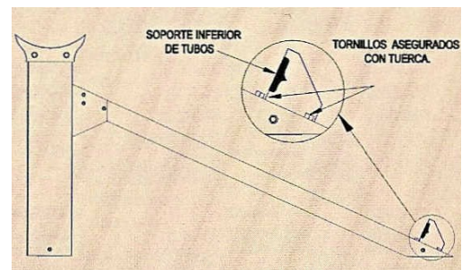
Figura 5 soporte sujeta tubos de vacío
