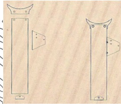
Figura 1 armado de patas
