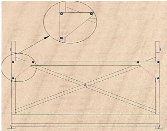
Figura 6 escuadras y travesaños
