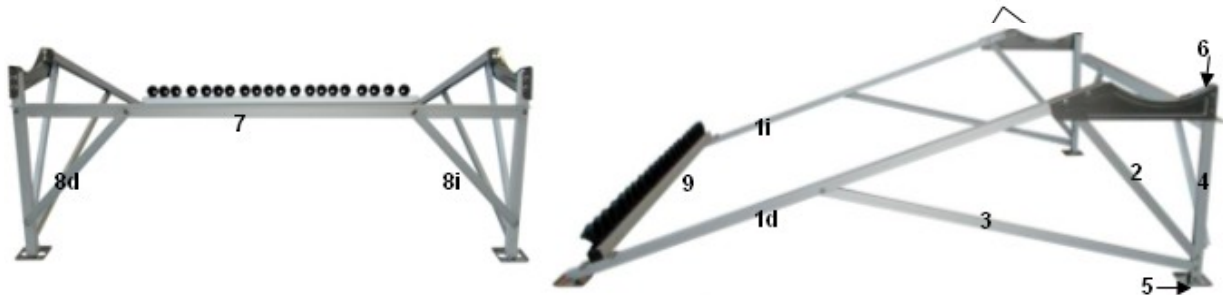
Figura 1 Armado de estructura de soporte
