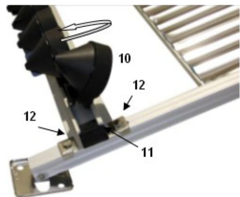
Figura 3 Sujetadores de tubos de vacío
