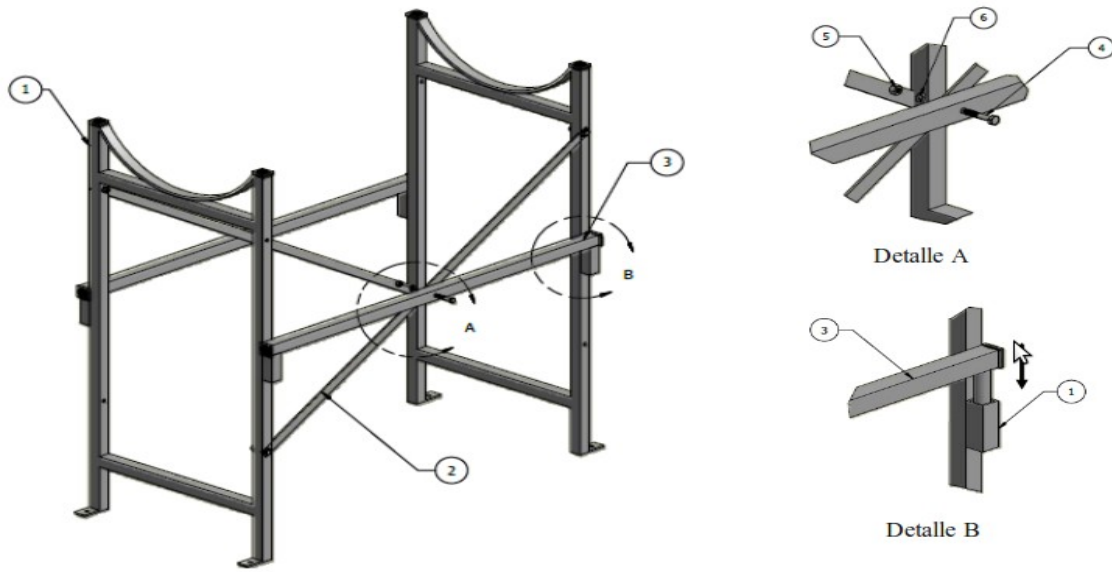
Figura 1 estructura de soporte
