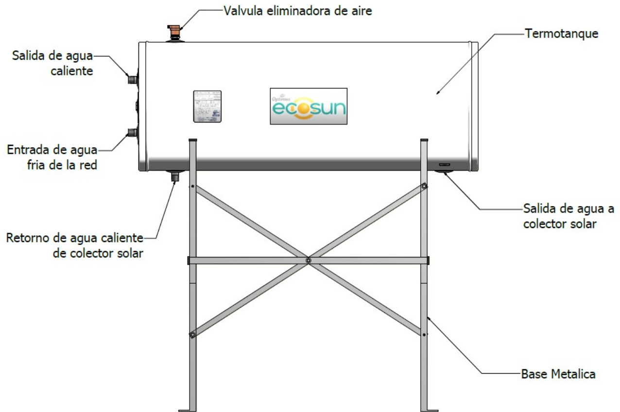
Figura 2 colocación del termotanque en la estructura de soporte
