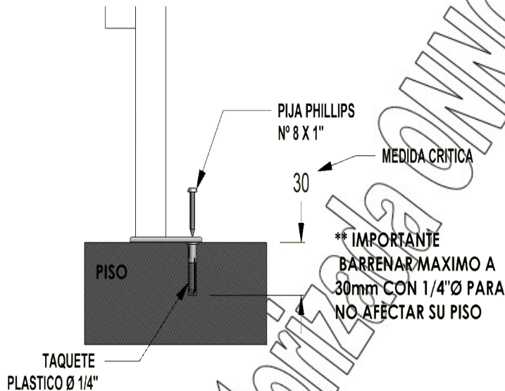
Figura 3 anclaje de la estructura de soporte
