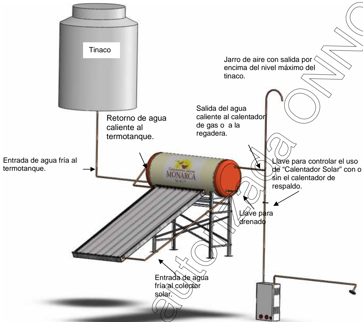
Diagrama de instalación hidráulica
