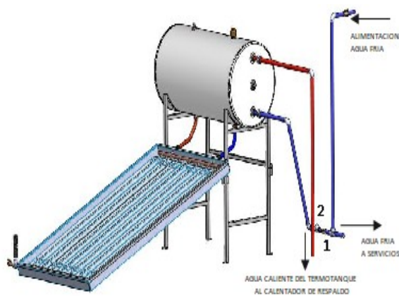
Figura 5 Conexiones del termotanque
