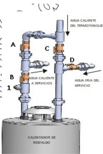
Figura 7 Conexión hidráulica del “Calentador Solar”
