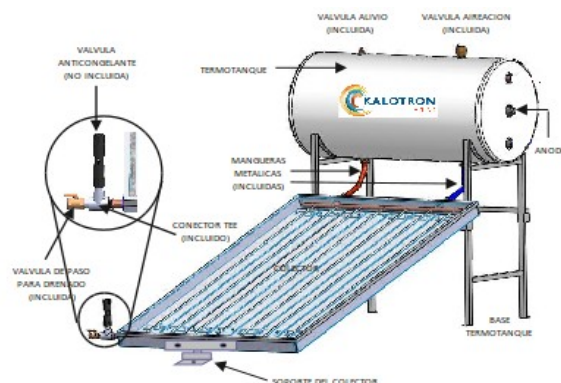
Figura 6 Protección anticongelante
