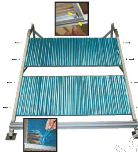
Figura 2 Colocación de reflectores
