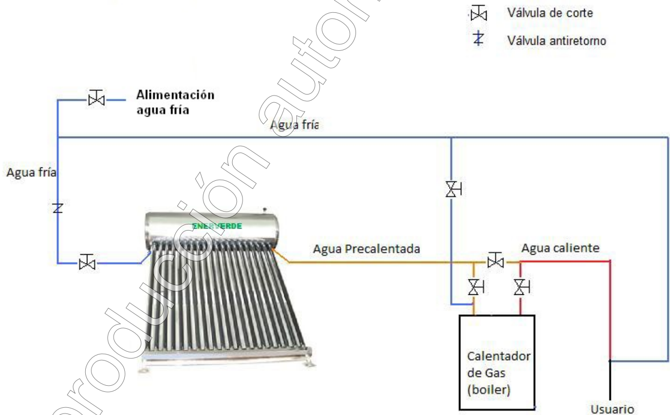
Figura 5 Instalación hidráulica
